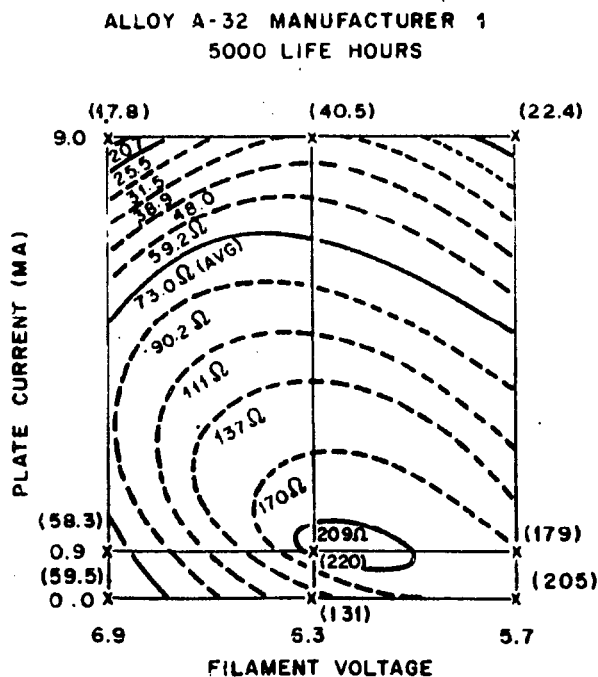
Fig. VI - INTERFACE READING CONTOURS-TRIODES
